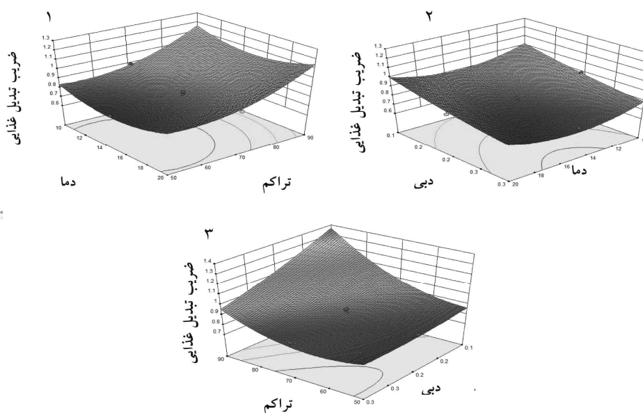
شکل ۲- تغییر در ضریب تبدیل غذایی ماهی قزل‌آلای رنگین‌کمان در اثر فاکتورهای مورد مطالعه. (۱): تأثیر دماهای مختلف و تراکم‌های مختلف در ضریب تبدیل غذایی، (۲): تأثیر دماهای مختلف و دبی‌های مختلف در ضریب تبدیل غذایی، (۳): تأثیر دبی‌های مختلف و تراکم‌های مختلف در ضریب تبدیل غذایی. متغیرهای دیگر در مقادیر متوسط ثابت در نظر گرفته شدند.
